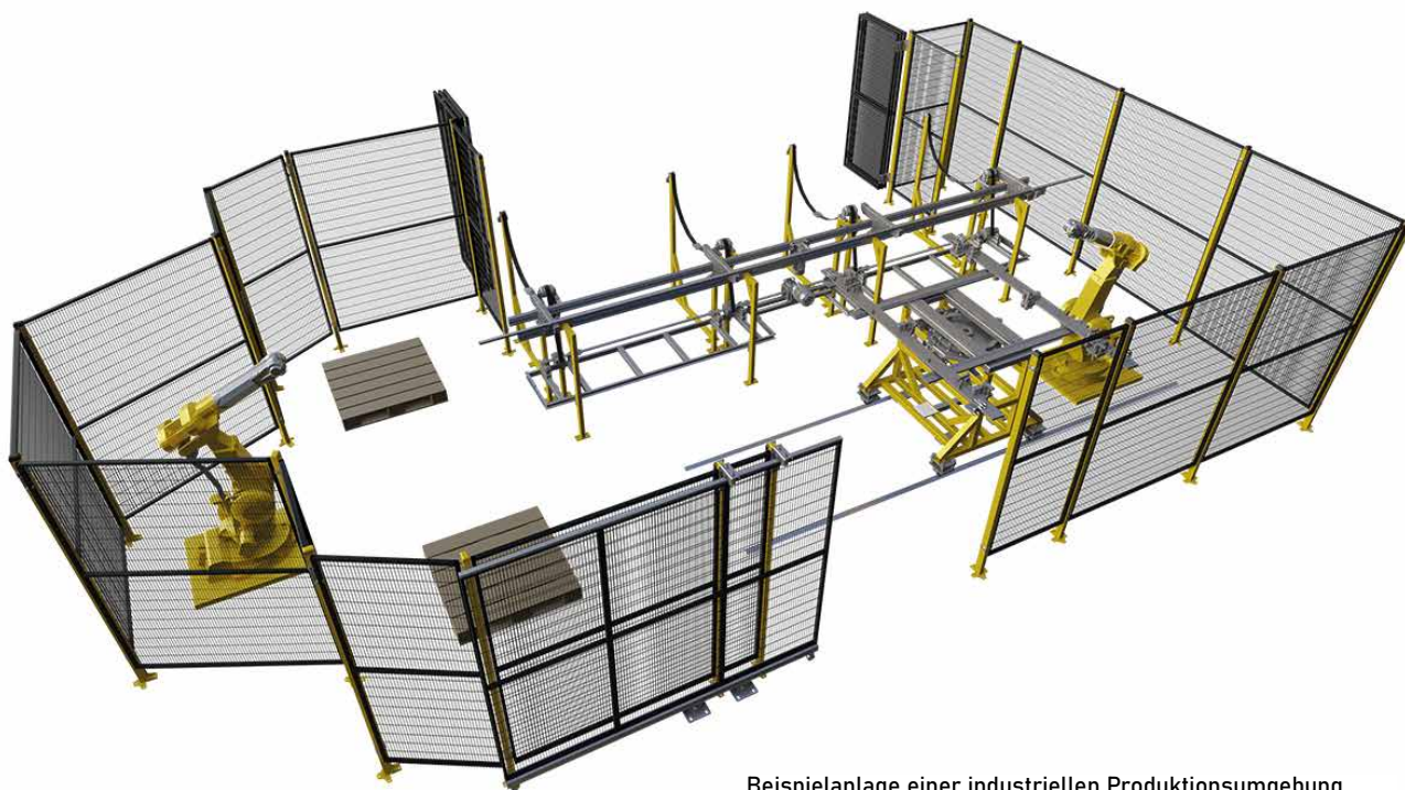
Beispielanlage einer industriellen Produktionsumgebung
